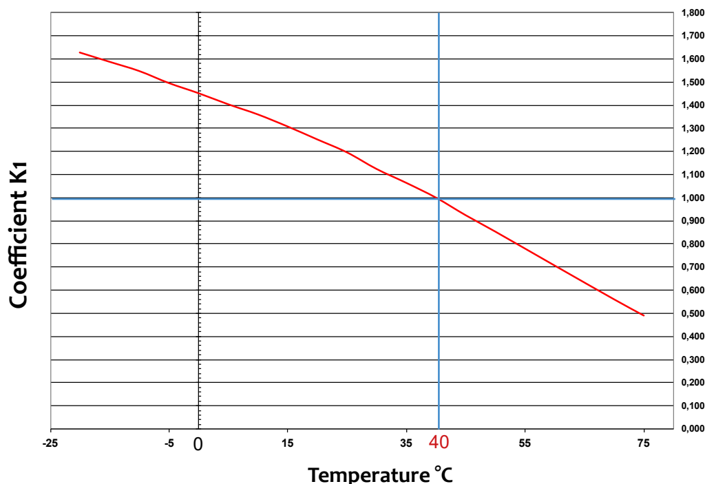
Temperature Factor K1 / Fattore Temperatura K1
